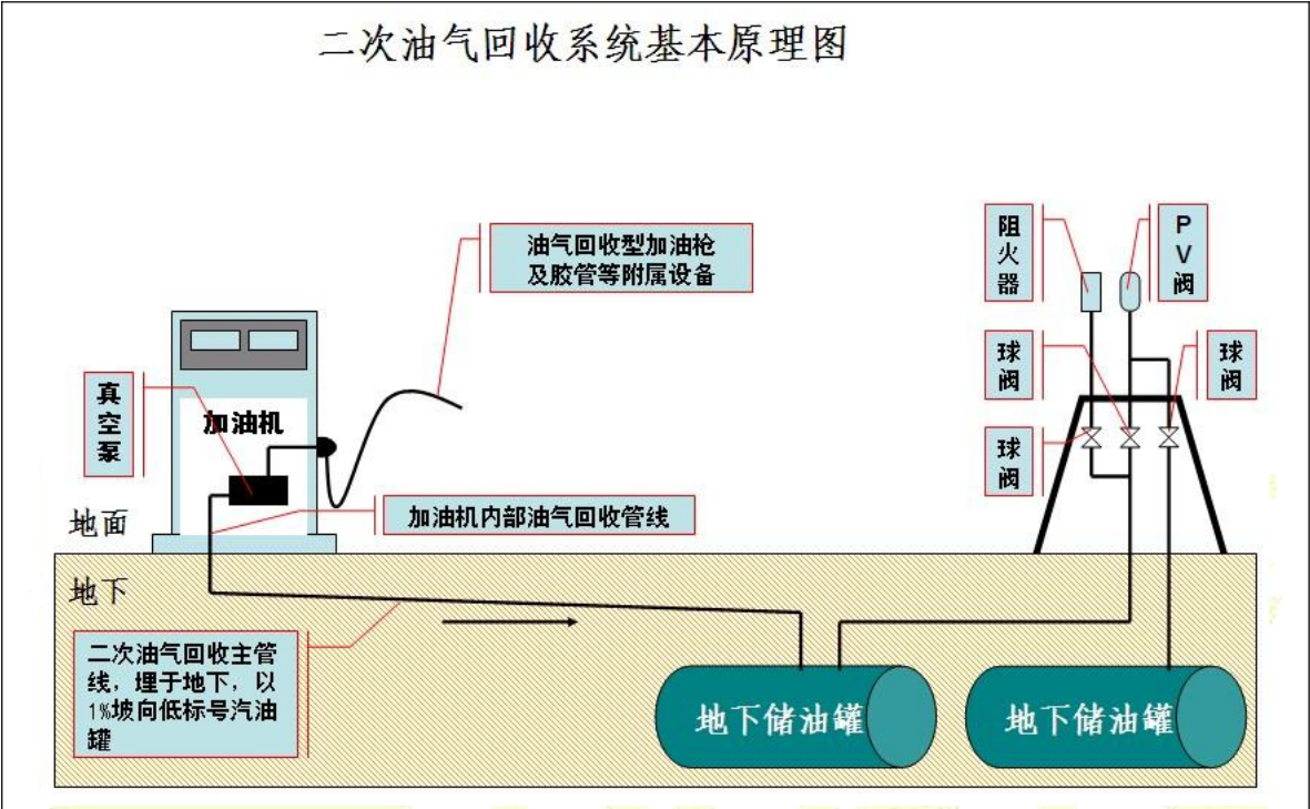
图 2.5-5 二次油气回收系统基本原理图
