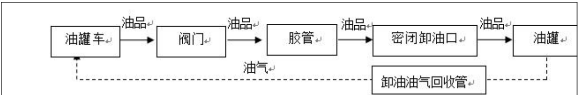
图 2.5-3 汽油卸油工艺流程图
