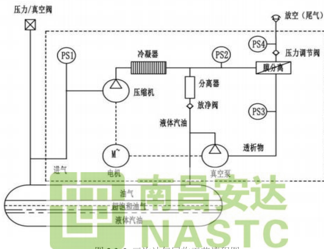
图 2.3-5 三次油气回收工艺流程图
