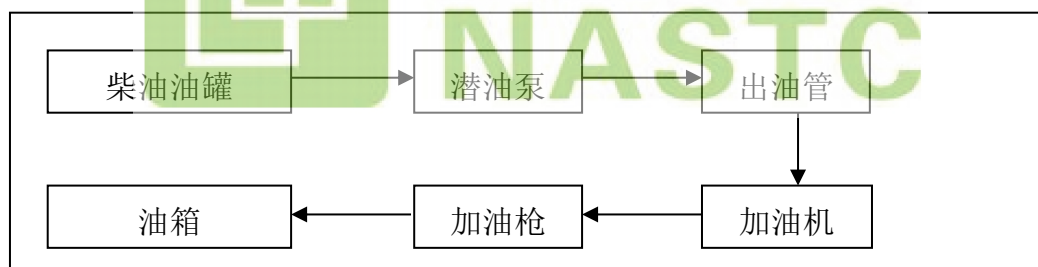
图 2-4 柴油加油工艺流程示意图
