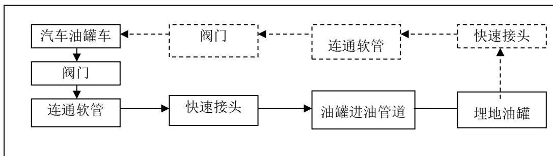
图 2-1 汽油卸油工艺流程示意图
