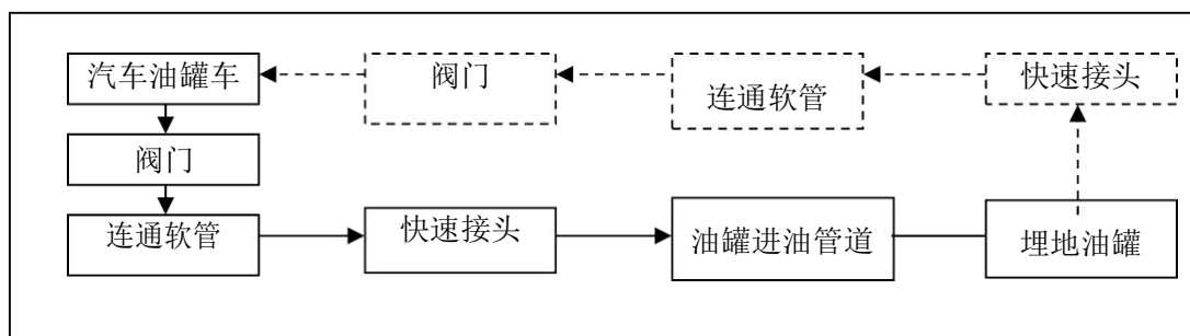
图 2-1 汽油卸油工艺流程图
