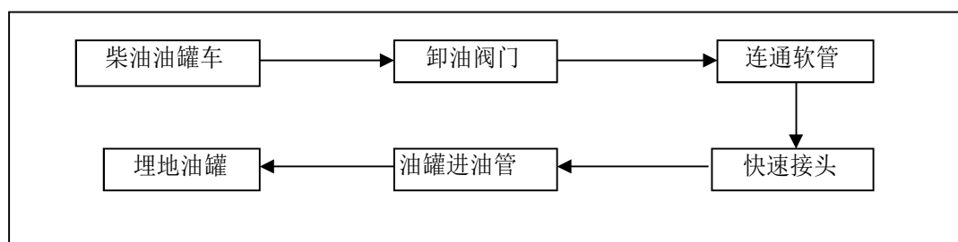
图 2-2 柴油卸油工艺流程图
