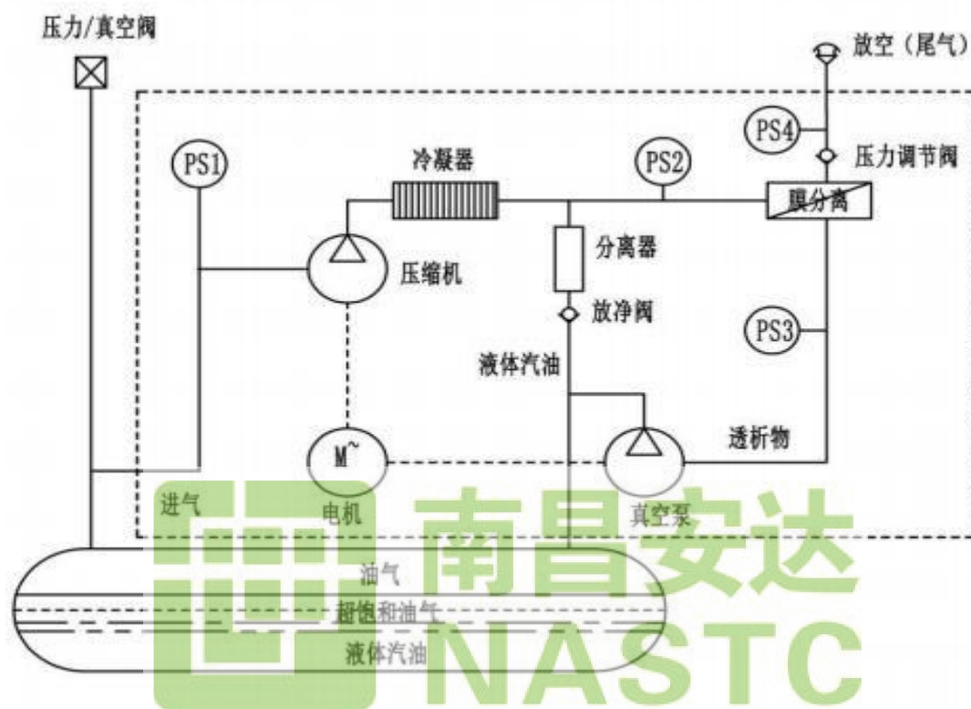
图 2-5 三次油气回收工艺流程图
