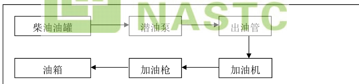
图 2-4 柴油加油工艺流程示意图
