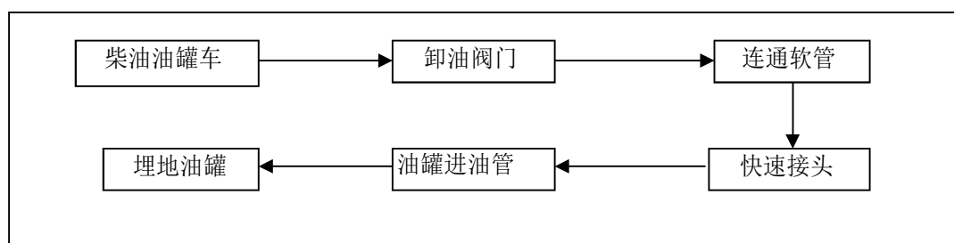
图 2-2 柴油卸油工艺流程示意图
