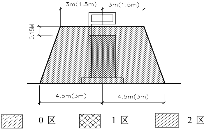
图 3.10-2 汽油加油机爆炸危险区域划分
