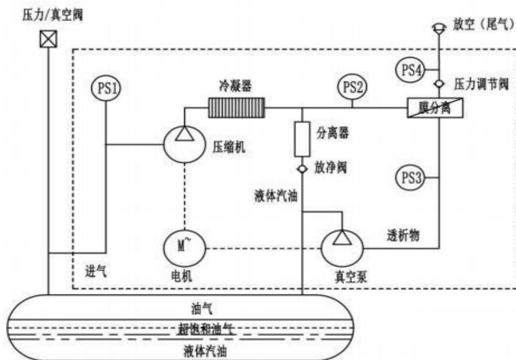
图 2-5 三次油气回收工艺流程图
