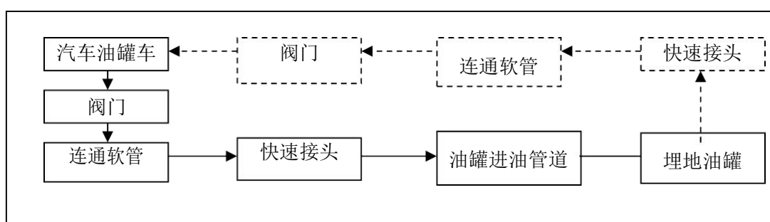
图 2-1 汽油卸油工艺流程图
