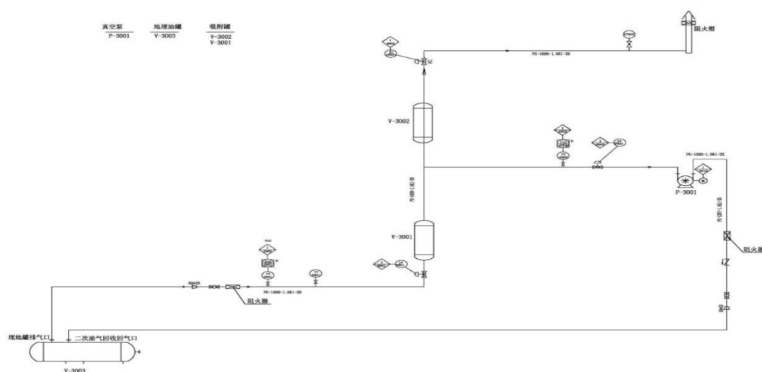
图 2.3-5 三次油气回收工艺流程图
