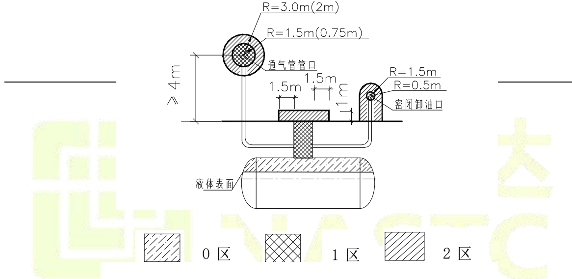
图3.9-1 埋地卧式汽油储油罐爆炸危险区域划分
