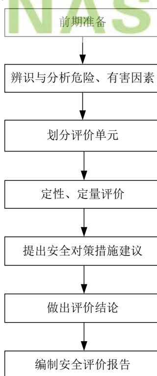
图 1.5-1 安全评价程序方框图
