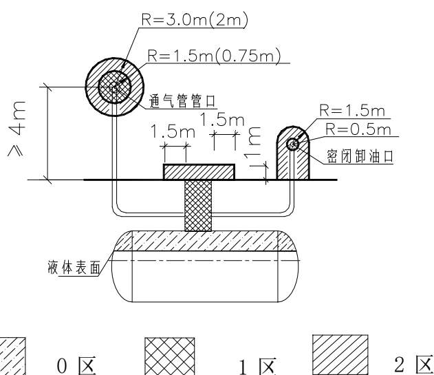
图3.9-1 埋地卧式汽油储罐爆炸危险区域划分
