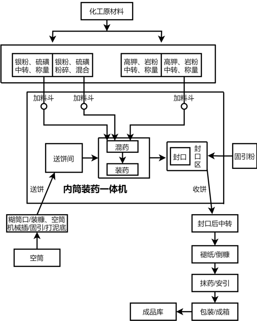
图 2-1：C 级爆竹类（单个白药炮）产品生产工艺流程
