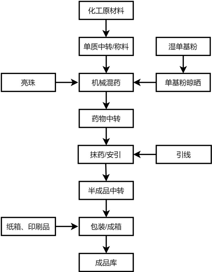
图 2-2：C 级玩具类(玩具造型)产品生产工艺流程
