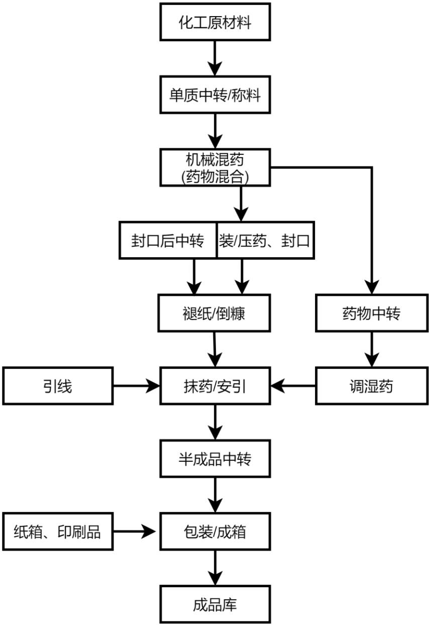
图 2-3：C 级喷花类(闪光炮)产品生产工艺流程
