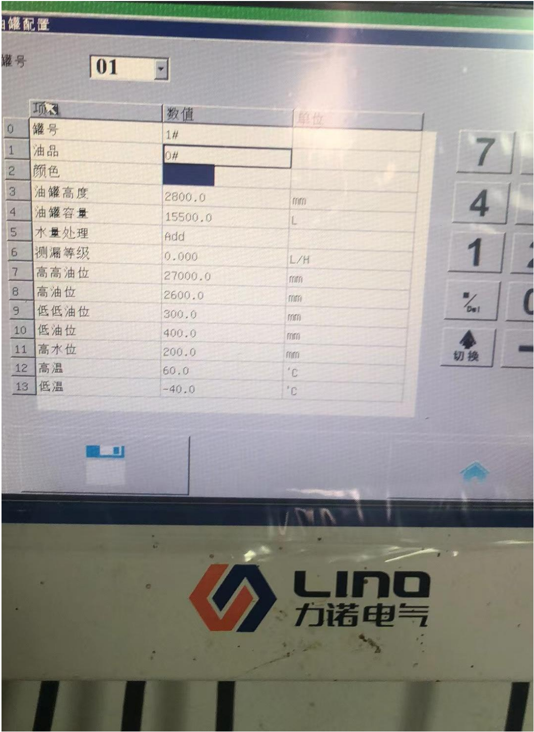
液位测量容积图片
