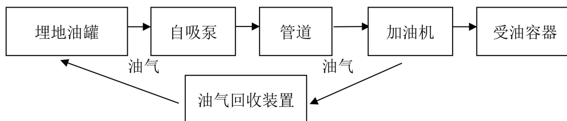
图 2.2-2 汽油加油工艺流程图
