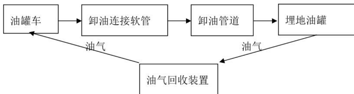
图 2.2-1 汽油卸油工艺流程图
