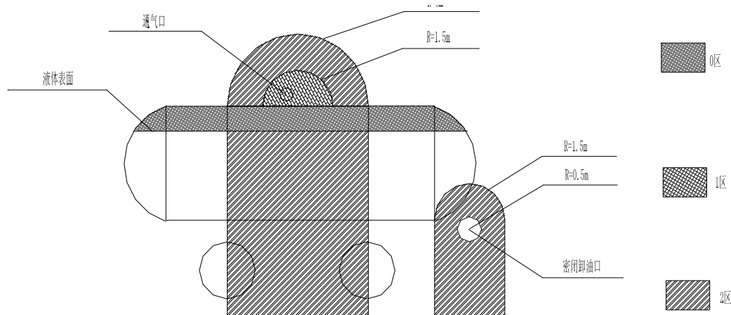
图 3.3-2 油罐车卸油爆炸危险区域划分
