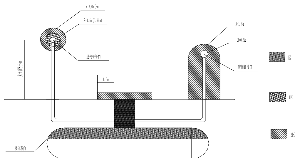
图 3.3-3 埋地油罐爆炸危险区域划分
